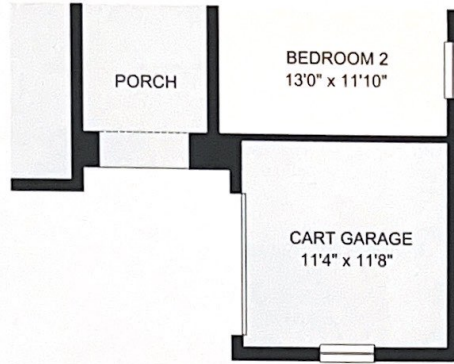
Optional Cart Garage
